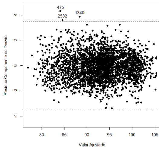
Figura 6.6: Gráfico dos valores ajustados pelo resíduo componente do desvio.
