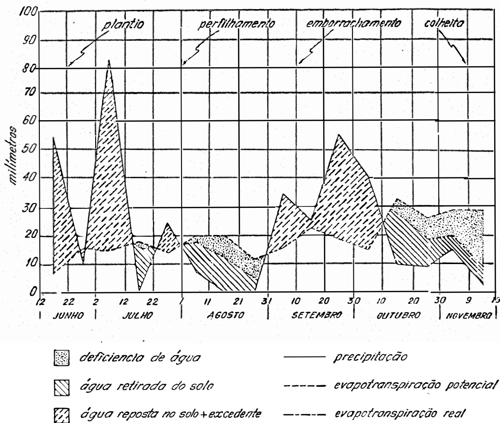
Figura 1 - Cursos (semeadura a colheita do trigo) da precipitação, evapotranspiração potencial e real, disponibilidades normais de água no solo, segundo o método do balanço hídrico de Thornthwaite e Mather, 1955.
