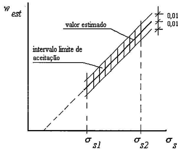
FIGURA 4.4 - Esquema do intervalo limite de aceitação ( \pm 0,01 mm)
