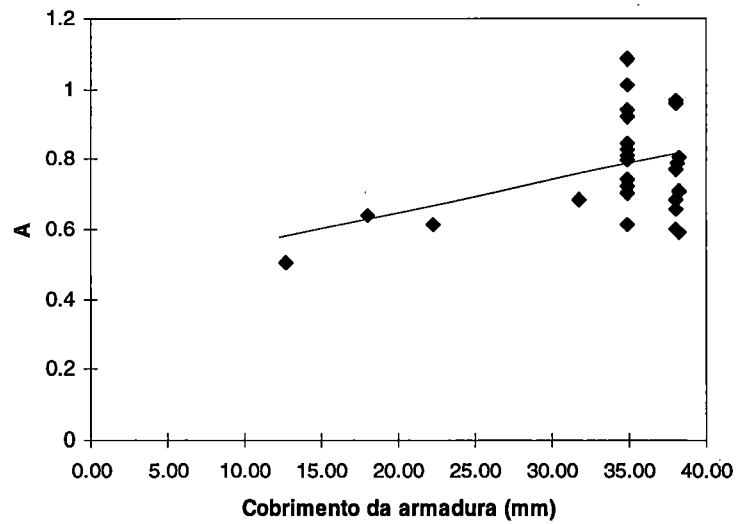
FIGURA 3.7 - Relação de A com o cobrimento de concreto da armadura (34 vigas)
