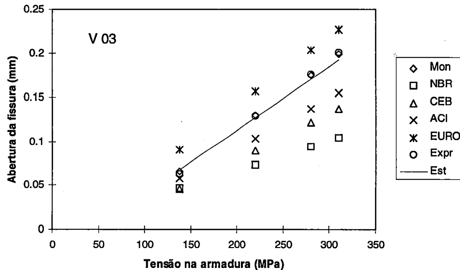
FIGURA 4.3 - Valores das aberturas das fissuras definidos pelas expressões propostas em relação aos valores da expressão estimada para a viga V 03.
