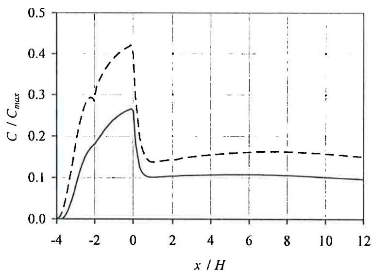
Figura 4.36: Perfis longitudinais de concentração relativa observados junto à superfície do túnel de vento. A linha pontilhada é determinada pela média da concentração somada a três vezes o desvio padrão.
