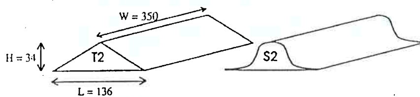
Figura 2.5: Obstáculos bidimensionais utilizados nos ensaios experimentais de Costa; Riethmuller; Borrego (1993). Dimensões em milímetros.
