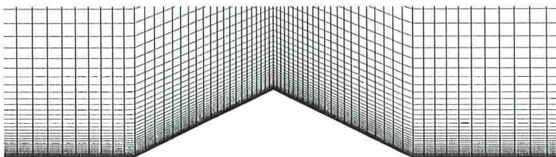
Figura 4.6: Malha gerada para simulação do escoamento bidimensional sobre a montanha de seção triangular, com refinamento em progressão geométrica na parede e no topo da montanha. Detalhe nas proximidades da montanha.
