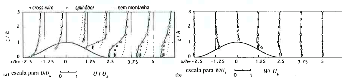
Figura 2.12: Distribuição das componentes longitudinal e vertical da velocidade média, no plano central do túnel de vento. Ishihara; Hibi; Oikawa (1999)
