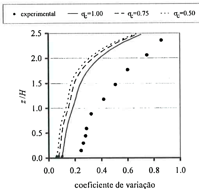
Figura 4.31: Influência do número de Prandtl turbulento \sigma_t no cálculo da variância da concentração, para constante C_G=1,0 .
