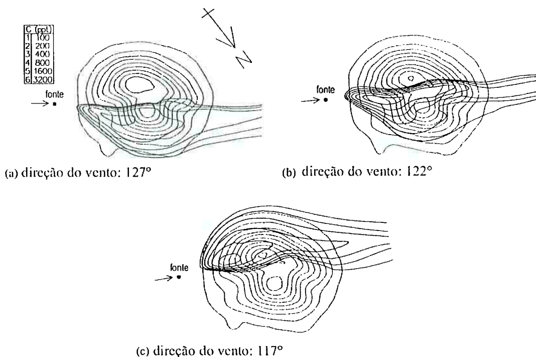
Figura 2.42: Influência da direção do vento sobre os resultados numéricos obtidos para o campo de concentrações. Apsley (1995)
