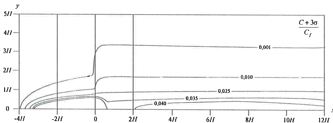
Figura 4.37: Linhas de concentração média mais três vezes o desvio padrão, normalizada pela concentração da fonte.
