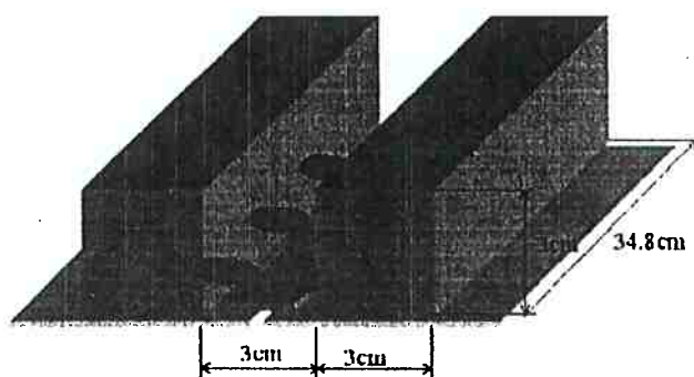
Figura 2.46: Configuração geométrica utilizada para representar o vale (street canyon) Sagrado et al. (2002)
