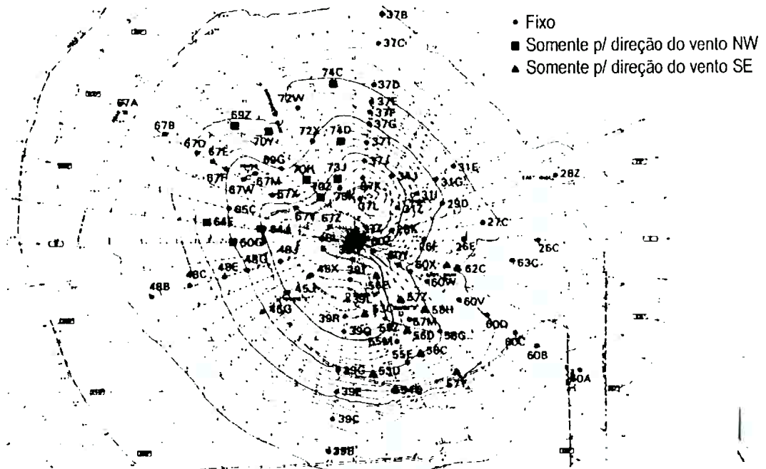
Figura 2.27: Posições dos amostradores de gases. Lavery et al. (1981).
