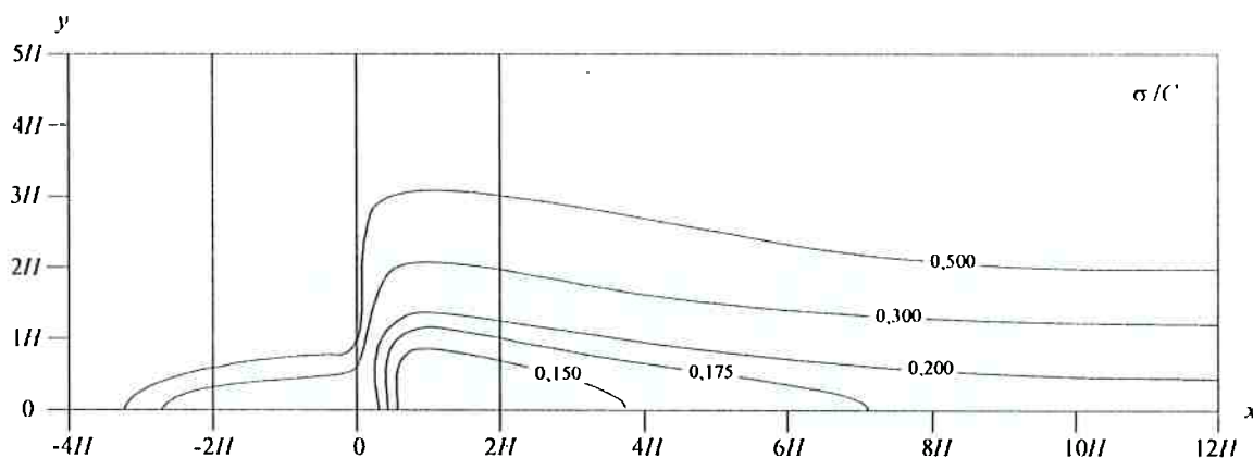
Figura 4.29: Linhas de coeficiente de variação constante para a superfície do túnel de vento e da montanha. C_G=0,5 e \sigma_c=0,75 .
