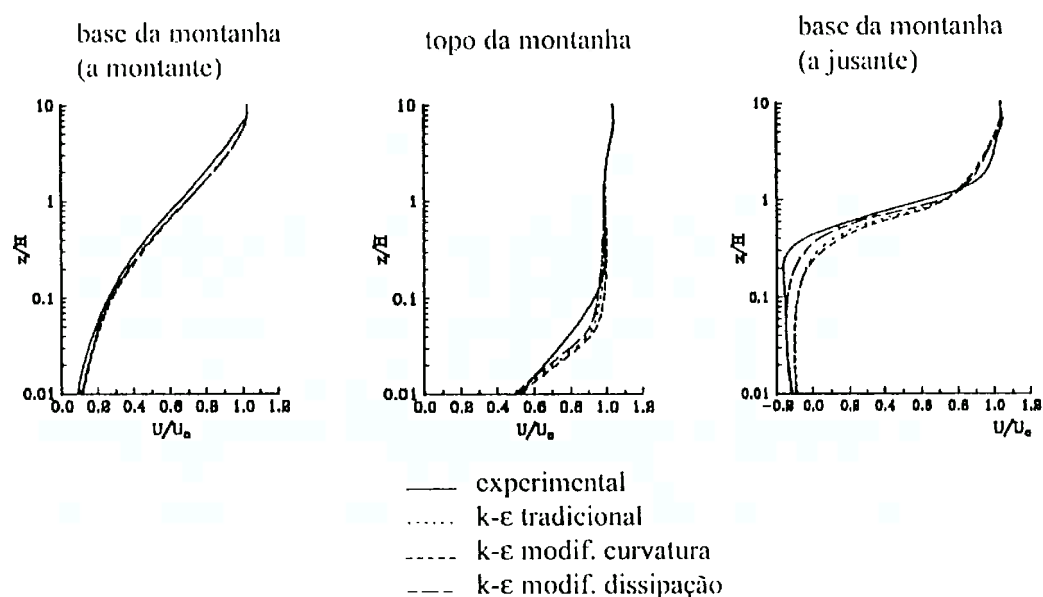
Figura 2.35: Comparação dos perfis verticais de velocidade experimental e numérico a montante, no topo e a jusante da montanha. Apsley (1995)
