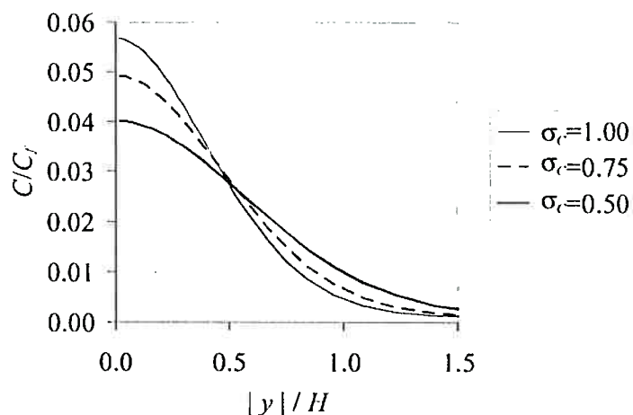
Figura 4.27: Perfil transversal de concentração relativa (à concentração da fonte) para o escoamento B – camada limite atmosférica simulada em túnel de vento – na posição 4H . Influência do número de Schmidt turbulento \sigma_C .
