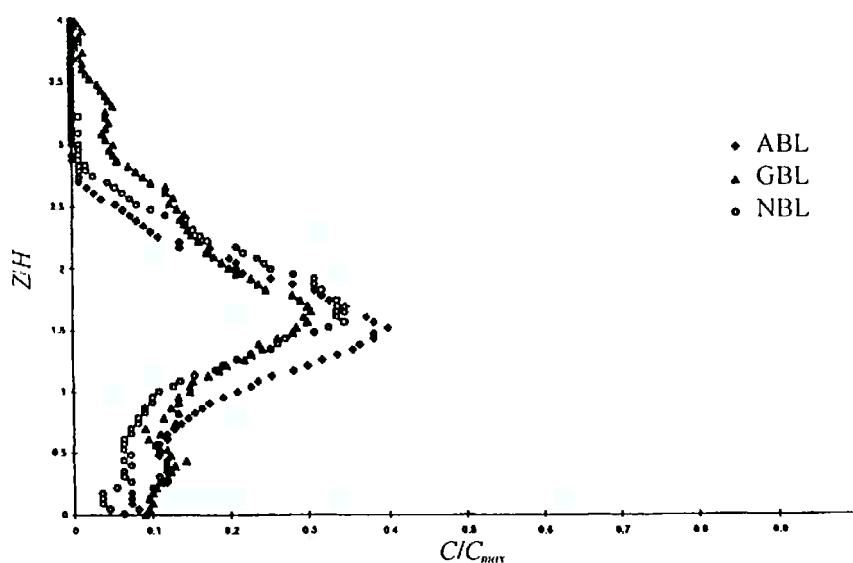
Figura 2.17: Perfis verticais de concentração para os três diferentes perfis de velocidade e intensidade de turbulência a montante, para a posição 2H e fonte de emissão com altura 1/2H . Chatzipanagiotidis; Olivari (1996)
