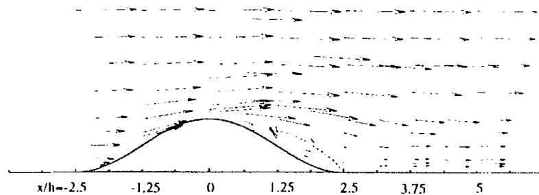
Figura 2.11: Vetores velocidade média no plano central do túnel de vento. Ishihara; Hibi; Oikawa (1999)
