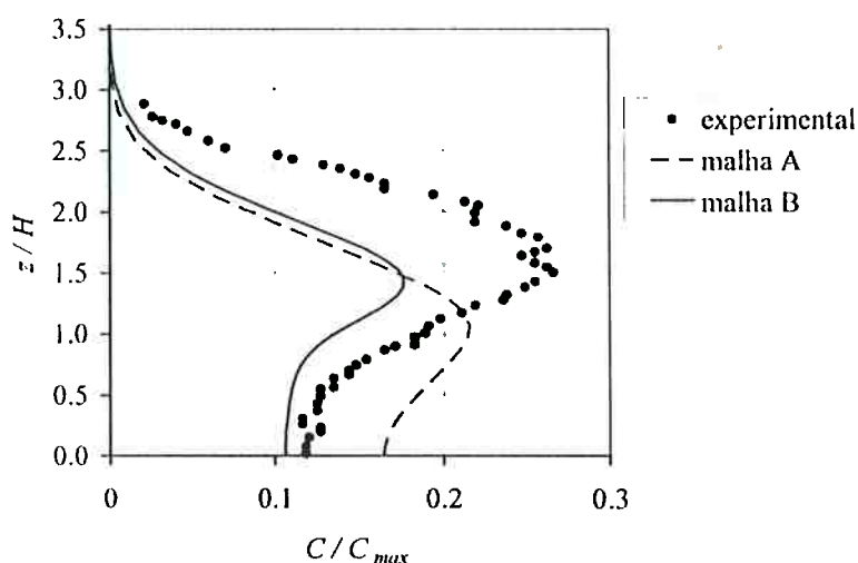
Figura 4.21: Comparação dos perfis verticais de concentração relativa C/C_{max} para o escoamento B, na posição x=4H , obtidos numericamente com os disponíveis na no trabalho de Chatzipanagiotidis; Olivari (1996).
