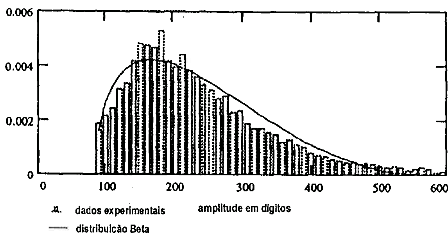
Figura 4.34: Distribuição da densidade de probabilidade juntamente com função Beta truncada convenientemente ajustada por Chatzipanagiotidis; Olivari (1996). Posição x=4H e z=1,5H .
