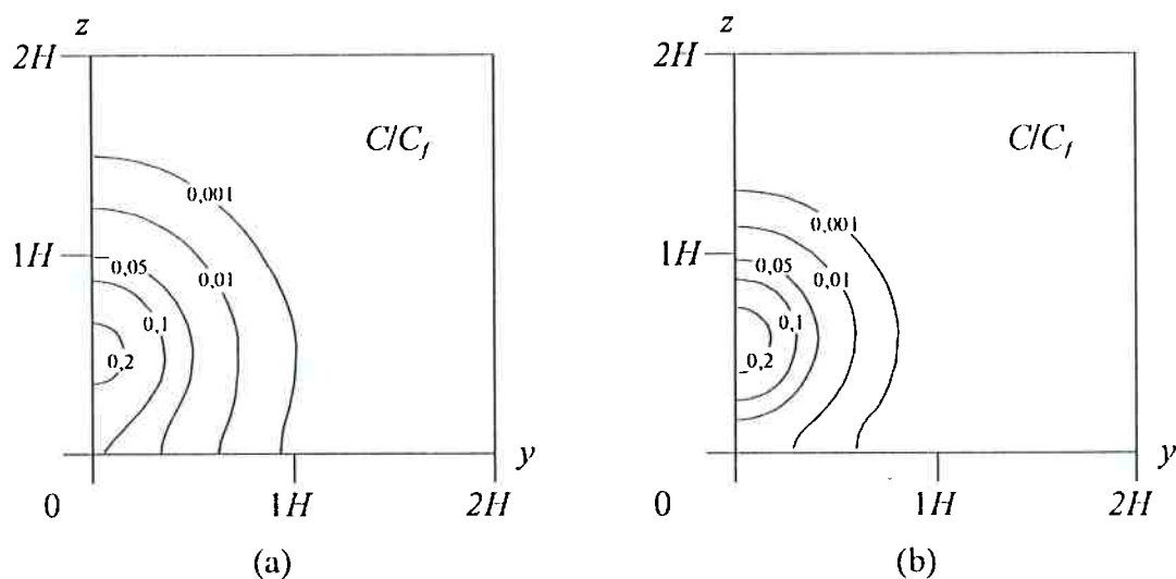
Figura 4.18: Linhas de isoconcentração relativa C/C_f para a seção x=-3H . (a) malha A (mesma malha utilizada na solução do escoamento); (b) malha B (malha refinada nas proximidades da fonte de despejo).
