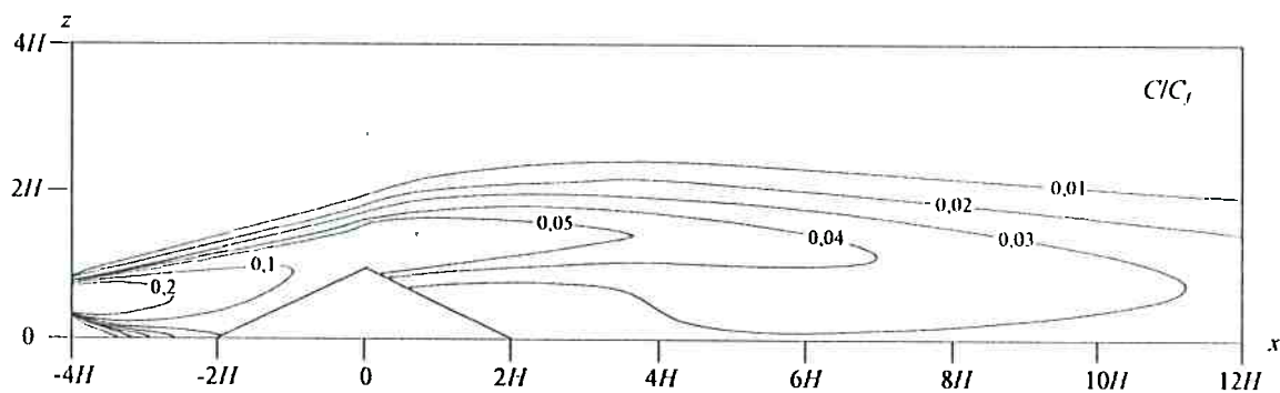
Figura 4.23: Linhas de iso-concentração média para o plano central do túnel de vento: y=0H .
