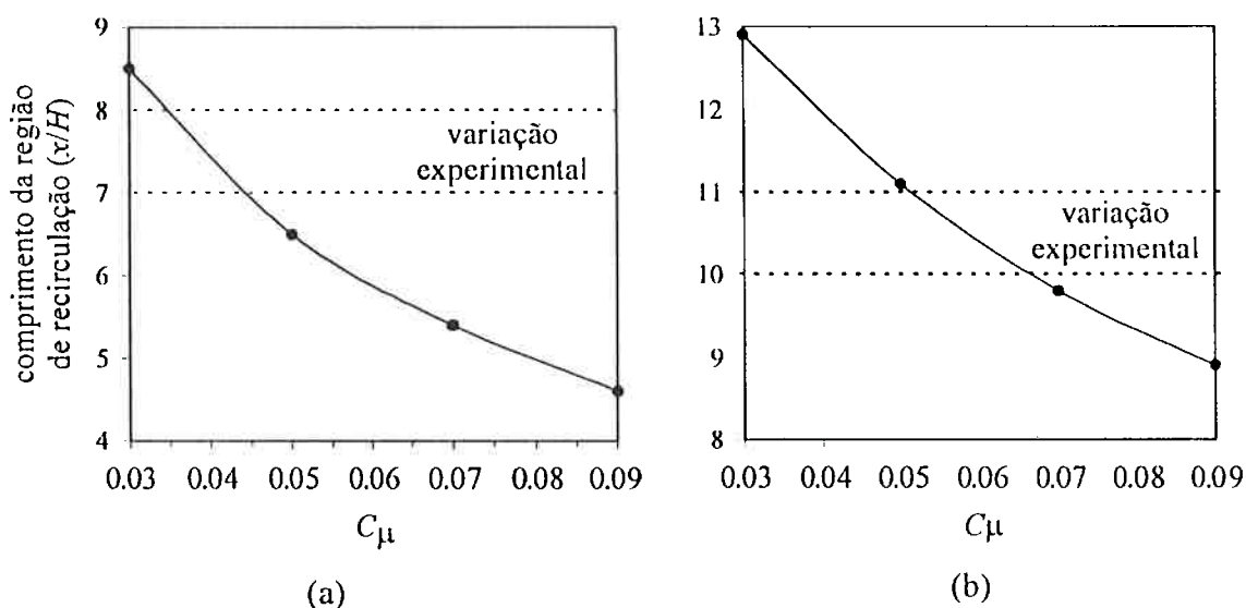
Figura 4.9: Comprimento da região de recirculação obtido numericamente em função da constante C_\mu do modelo k-\epsilon ; (a) escoamento B; (b) escoamento N.
