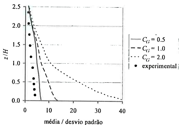
Figura 4.32: Perfil vertical da média da concentração sobre desvio padrão.
