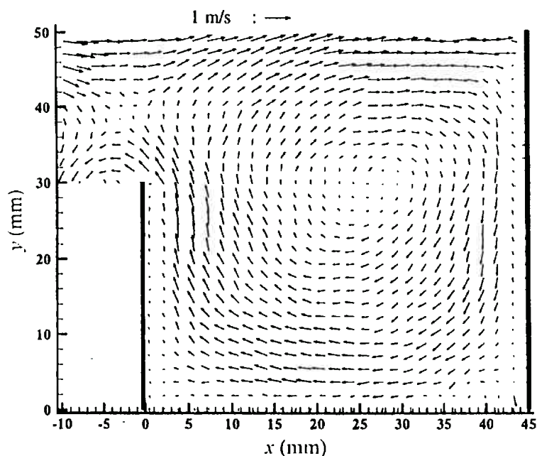
Figura 2.21: Campo de velocidades formado no interior do vale obtido com a técnica experimental PIV – particle image velocimetry – Gerdes; Olivari (1999).
