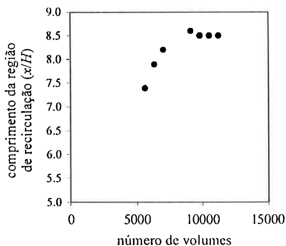
Figura 4.8: Influência da malha sobre o comprimento da região recirculação formada a jusante da montanha de seção triangular.
