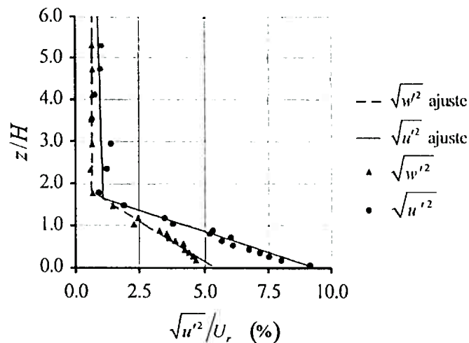
Figura 4.4: Perfis verticais das flutuações turbulentas para o escoamento N (camada limite de baixa turbulência desenvolvida na superfície do túnel de vento). As linhas são ajustes para retas.
