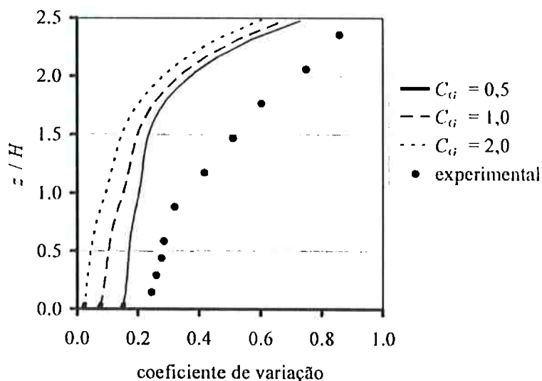
Figura 4.30: Influência da constante C_G no cálculo do coeficiente de variação, para número de Schmidt turbulento \sigma_c = 0,75 .
