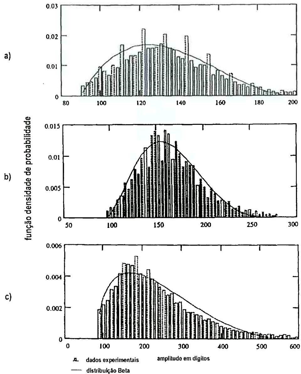
Figura 2.19: Distribuição da densidade de probabilidade juntamente com função Beta convenientemente ajustada para posições x=4H . a) z=0,15H b) z=0,36H c) z=1,51H . Chatzipanagiotidis; Olivari (1996)
