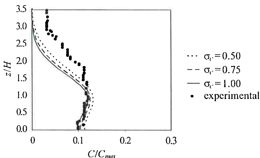
Figura 4.26: Comparação do perfil vertical de concentração relativa para o escoamento B – camada limite atmosférica simulada em túnel de vento – na posição 9H. Influência do número de Schmidt turbulento \sigma_t .
