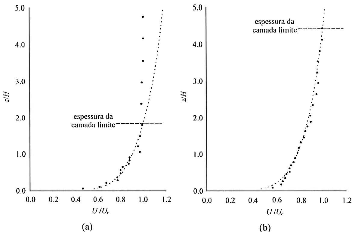
Figura 4.2: Perfis de velocidade N (a) e B (b) comparados com as respectivas relações de potência. Para o escoamento N \delta=60\text{mm}\cong 1,8H , enquanto que para o escoamento B \delta=150\text{mm}\cong 4,4H , onde H é a altura do obstáculo que simula a montanha.
