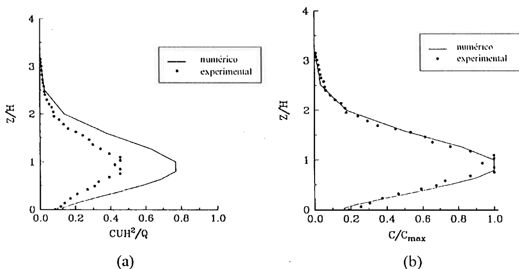
Figura 2.36: Comparação dos perfis verticais de concentração obtidos numericamente com os dados experimentais da literatura obtidos em túnel de vento: (a) concentração não normalizada; (b) concentração normalizada pela máxima observada na seção. Apsley (1995)
