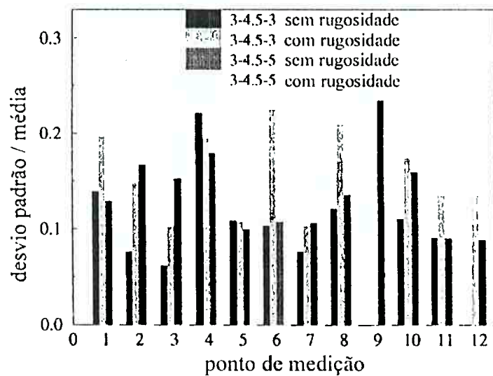
Figura 2.23: Desvio padrão normalizado pela média observado para diferentes posições e configurações geométricas do vale. Gerdes; Olivari (1999).
