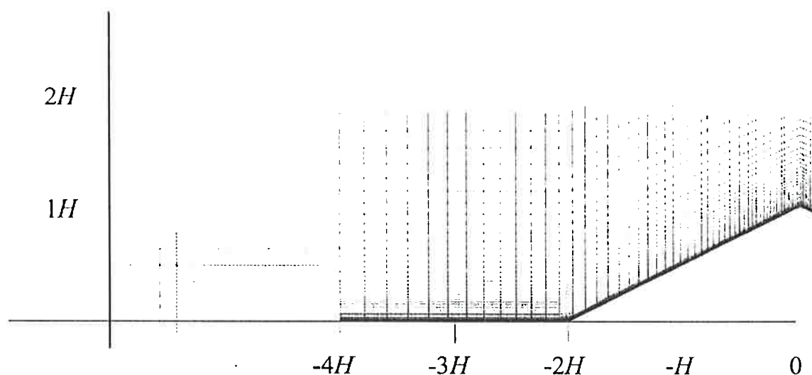
Figura 4.13: Malha A, refinada em progressão geométrica nas proximidades da parede e no topo da montanha, apropriada à solução do escoamento com o modelo de turbulência proposto por Lam; Bremhorst (1981). Vista ampliada nas proximidades da fonte: tubo de 10mm de diâmetro. Dimensões relativas à altura da montanha: H=34\text{mm} .
