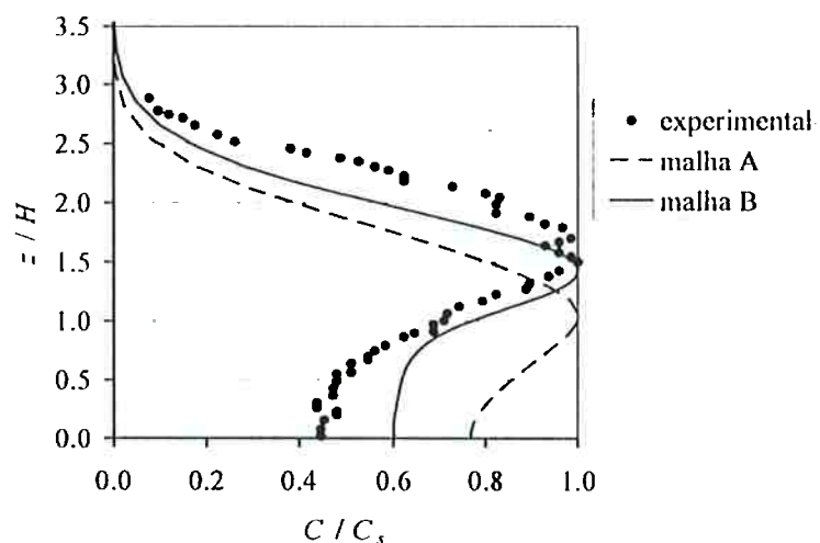
Figura 4.22: Comparação dos perfis verticais de concentração relativa C/C_s para o escoamento B, na posição x=4H , obtidos numericamente com os disponíveis na no trabalho de Chatzipanagiotidis; Olivari (1996).
