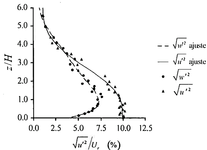
Figura 4.3: Perfis verticais das flutuações turbulentas para o escoamento B (camada limite atmosférica simulada). As linhas são ajustes para polinômios de grau cinco.
