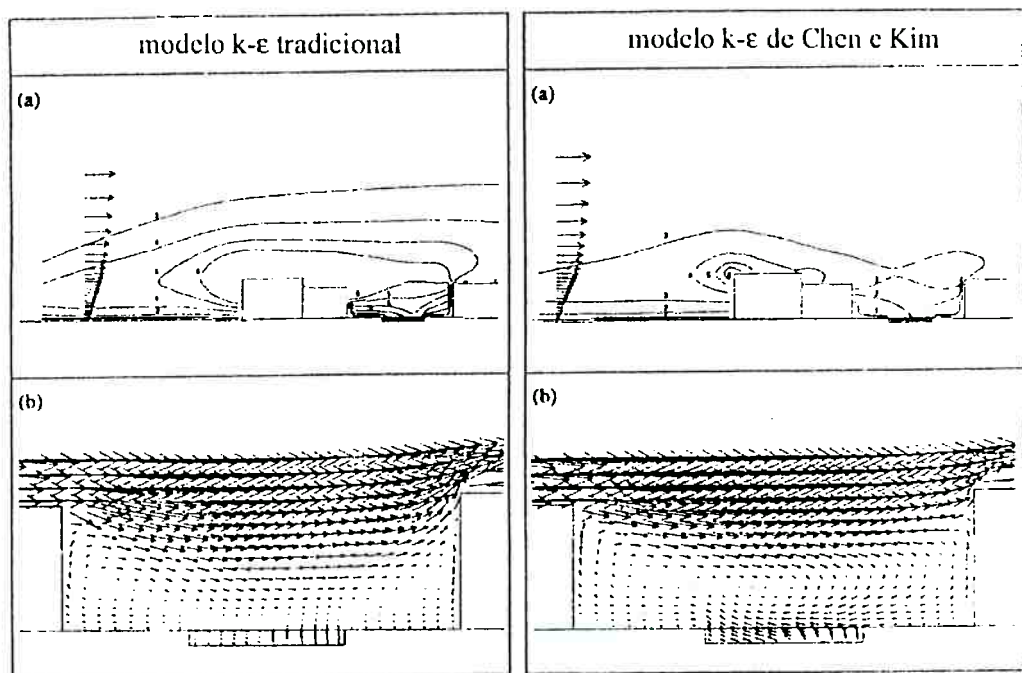
Figura 2.30: Comparação entre os modelos de turbulência: (a) isolinhas de energia cinética turbulenta e (b) vetores velocidade num plano vertical. Delaunay (1996)
