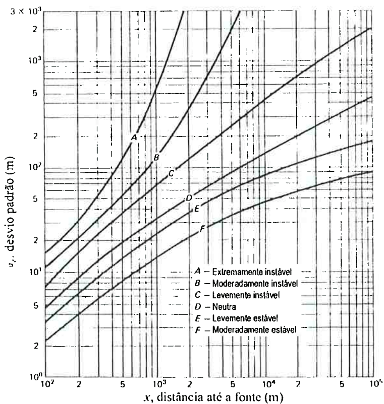
Figura 2.3: Desvio padrão \sigma_z para as diferentes classes de estabilidade Pasquill-Gifford. Seinfeld (1986).
