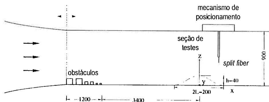
Figura 2.9: Desenho esquemático do túnel de vento. Ishihara; Hibi; Oikawa (1999)
