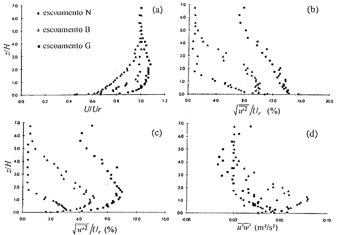
Figura 2.7: Medição dos perfis verticais de velocidade e flutuações turbulentas a montante da montanha (posição -6H ), relativos à velocidade de referência U_r=5\text{m/s} . Costa; Riethmuller; Borrego (1993)
