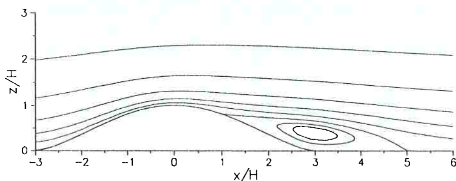
Figura 2.33: Resultado numérico de Apsley (1995) mostrando as linhas de corrente e a recirculação formada na parte posterior da montanha bidimensional de seção senoidal. Os dados experimentais utilizados para comparação foram obtidos em túnel de vento.
