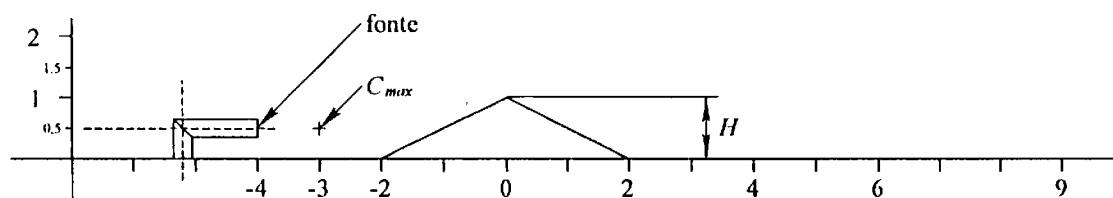
Figura 4.12: Posicionamento da fonte em relação à montanha e plano onde é avaliada a concentração de referência C_{max} . Dimensões relativas à altura da montanha bidimensional H=34\text{mm} .
