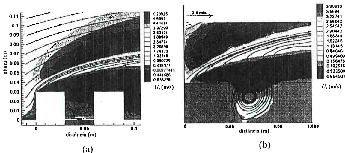
Figura 2.48: Comparação entre as linhas de corrente obtidas numericamente utilizando o código computacional Fluent 5.2 (a) e as linhas de corrente obtidas com a técnica experimental PIV (b). Sagrado et al. (2002) – figuras disponíveis apenas em escala de cinza, sem cores.
