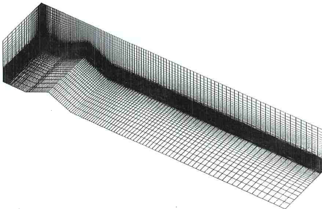
Figura 4.15: Malha utilizada no cálculo do campo de concentração. Dimensões: 836 mm × 136 mm × 170 mm – Volumes: 150 × 59 × 33
