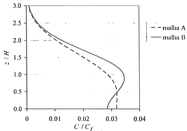
Figura 4.20: Comparação dos perfis verticais de concentração relativa C/C_f para o escoamento B, na posição x=9H , obtidos com malhas diferentes.
