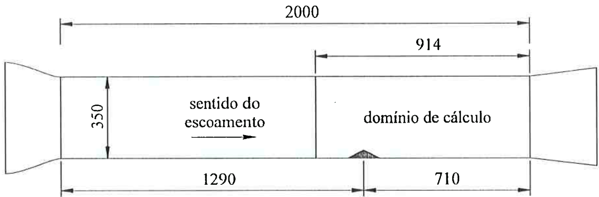
Figura 4.1: Dimensões do túnel de vento utilizado por Costa; Riethmuller; Borrego (1993). A região destacada é o domínio de cálculo da simulação numérica bidimensional - dimensões em milímetros.
