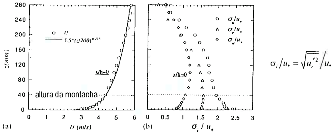
Figura 2.10: Perfis verticais de velocidade média (a) e intensidade de turbulência (b) – velocidade de atrito u_* = 0,212 \text{ m/s} . Ishihara; Hibi; Oikawa (1999)
