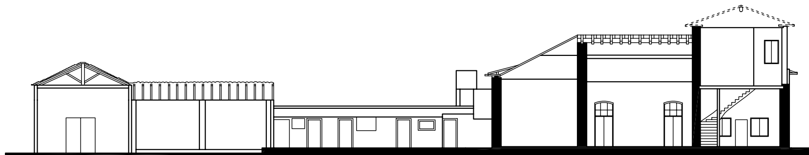
Corte AA
