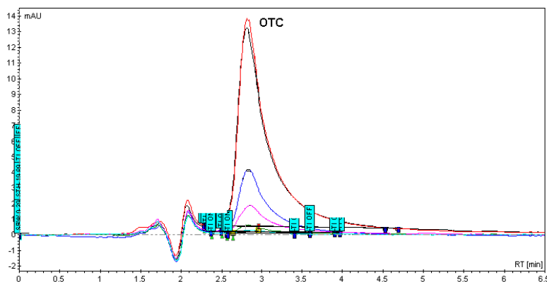
Figura 24. Cromatogramas sobrepostos para solo "M1" -OTC obtidos em pH 4,8, onde: C i OTC = 120 mg L -1 (preto), C i OTC = 60 mg L -1 (vermelho), C i OTC = 30 mg L -1 (azul), C i OTC = 20 mg L -1 (rosa).
