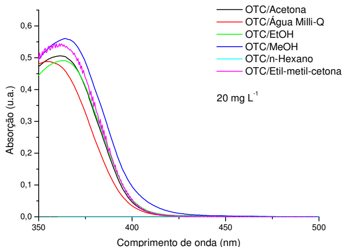
Figura 52. Sobreposição de espectros de absorção da OTC em diferentes solventes na região limite entre o UV e o Visível.
