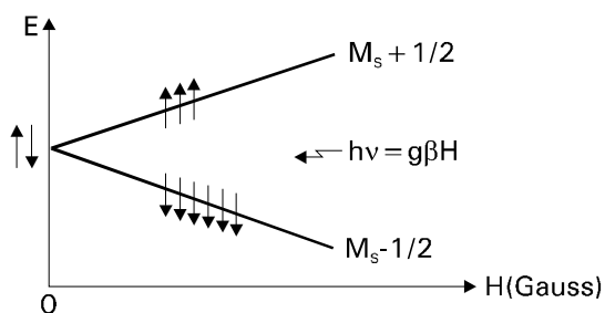
Figura 13. Representação esquemática do Efeito Zeeman.
