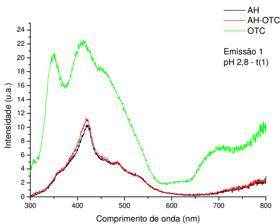
Figura 53. Sobreposição de espectros de Fluorescência no UV-Visível obtidos no modo de emissão, com ajuste de pH após período de interação de 24 h, com uma excitação em 240 nm.
