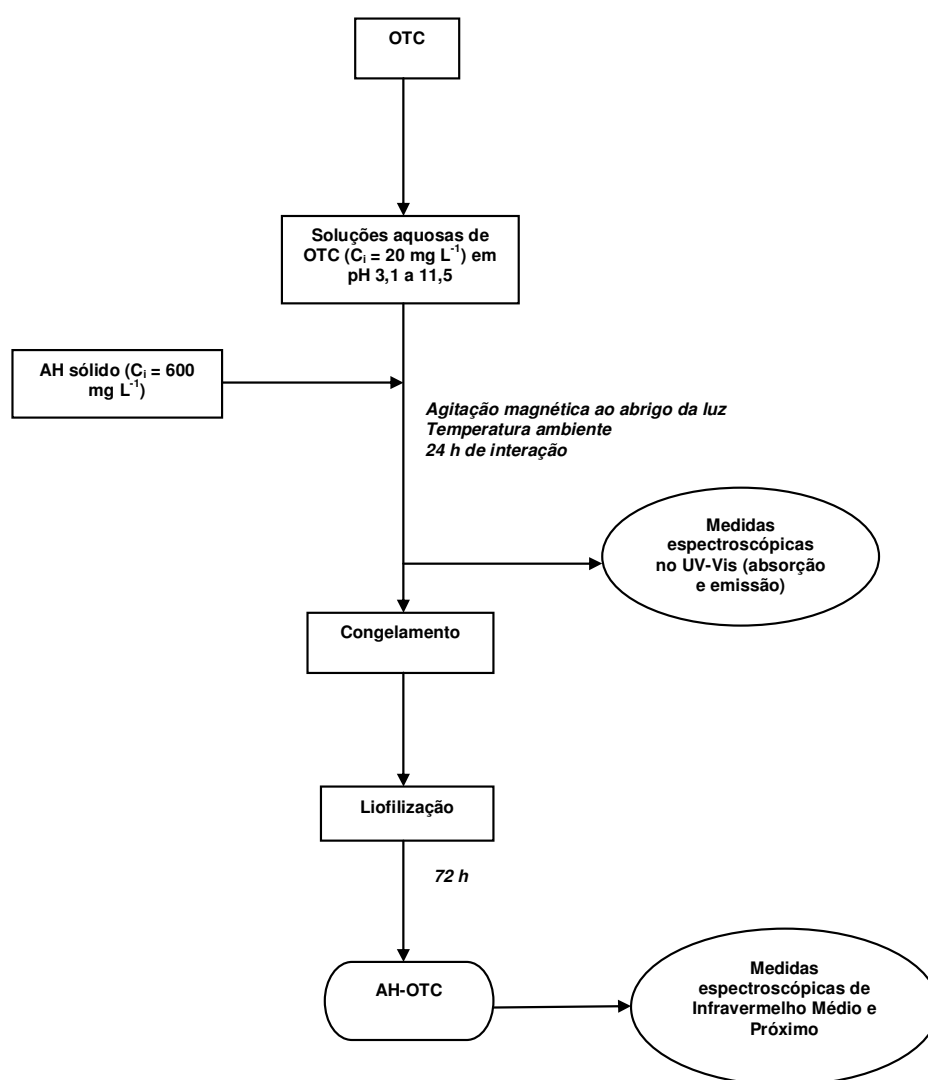
Figura 19. Fluxograma detalhado da ROTA 2 de preparo dos produtos de interação AH-OTC.
